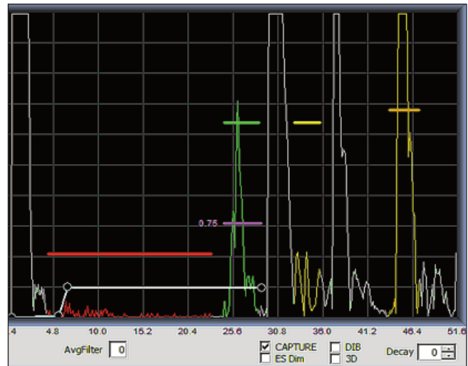
图为UT界面的A-扫描显示，图示通道1设置了1个界面面闸门和4个测量闸门
