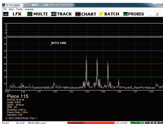
上图显示了 0.23mm, 0.2mm, 0.15mm 及 0.10mm 深的缺陷信号 (0.009", 0.008", 0.006" 及 0.004")
