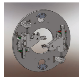
上图: 带有两个探头臂和探头的探头盘
